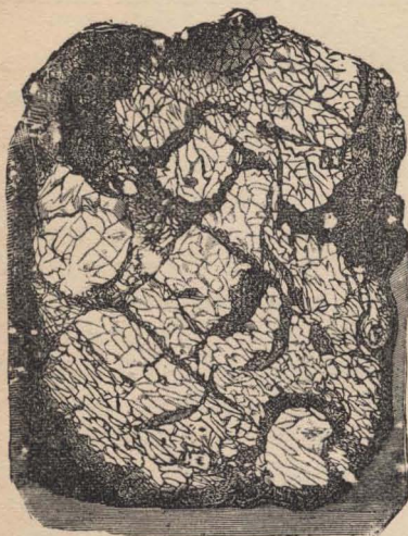
Aerolito.
