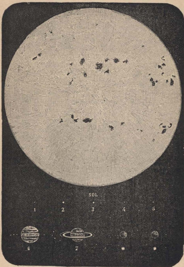
Tamaños comparados del Sol y de los planetas.
