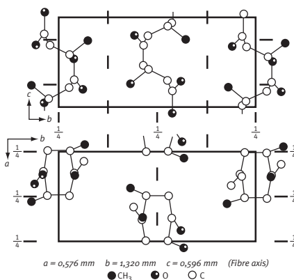
Figura 3: Celda unitaria de PHB.
