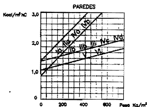
VALOR DE TRANSMITANCIA TÉRMICA K max. SEGUN ZONA BIOAMBIENTAL
