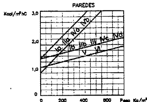
VALOR DE TRANSMITANCIA TÉRMICA K max. SEGUN ZONA BIOAMBIENTAL
