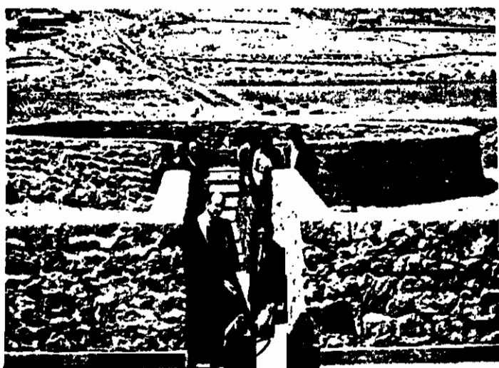
Bañadero de ovejas construido en Chaupí Rodeo, Jujuy, Argentina, como parte de una actividad del Proyecto Especial "Desarrollo Educativo Integrado de Zonas Límitrofes".
